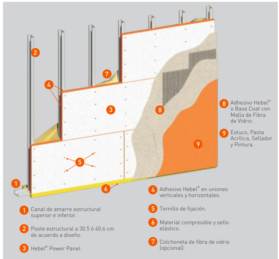
Fig. 22 Muro Exterior
